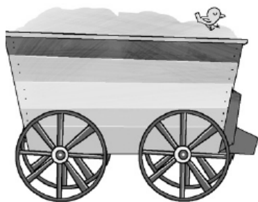
caro – carro
